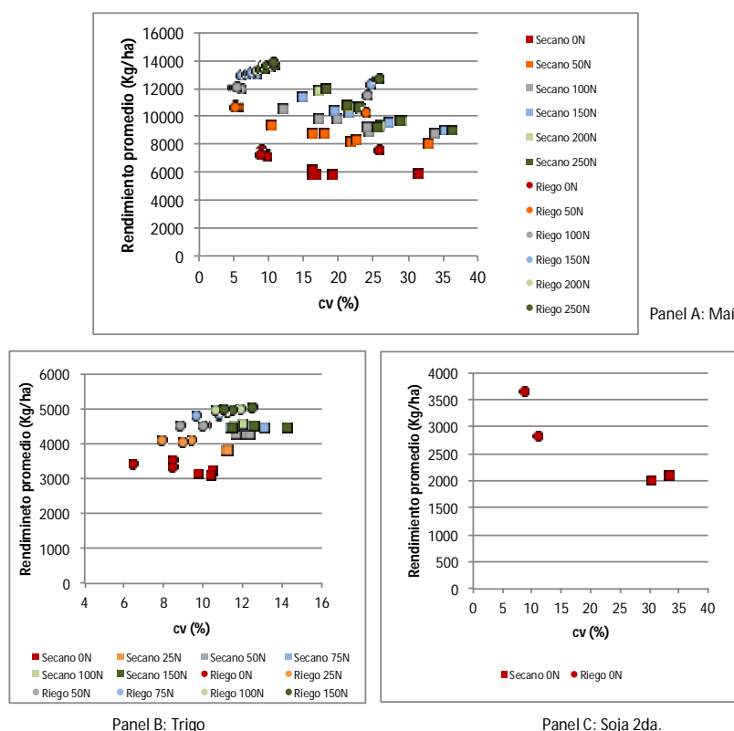
Figura 2. Rendimientos promedio y coeficiente de variación para maíz, trigo y soja 2 da en el Partido de Pergamino
